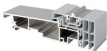
Seuil aluminium à rupture thermique
